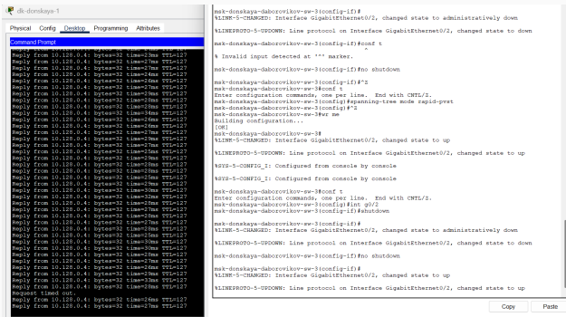
Figure 16: Отказоустойчивость протокола Rapid PVST+
