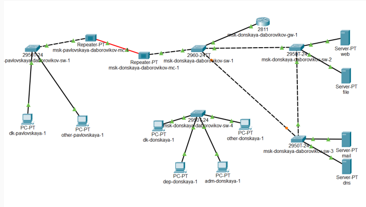
Figure 1: Логическая схема локальной сети с резервным соединением
