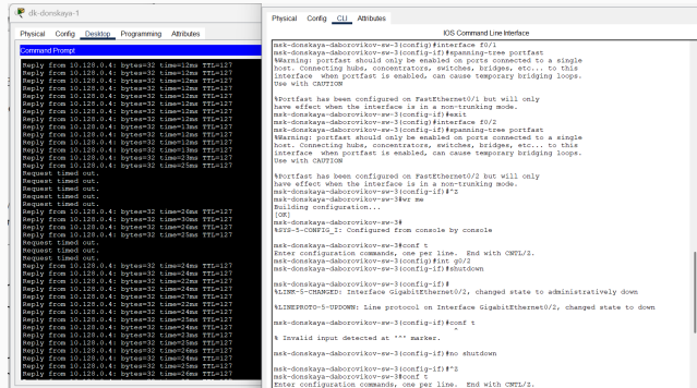
Figure 14: Отказоустойчивость протокола STP
