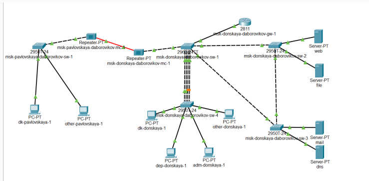
Figure 17: Логическая схема локальной сети с агрегированным соединением
