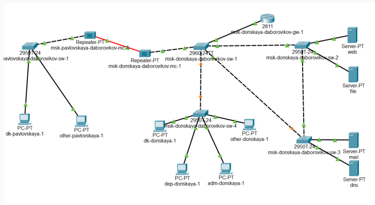
Figure 3: sw-1 и sw-4 через интерфейсы Fa0/23
